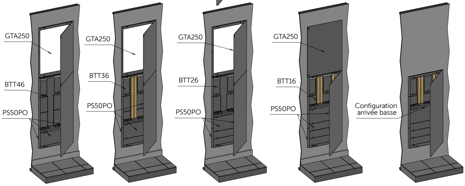
Exemple de mise en oeuvre avec GTA 250
